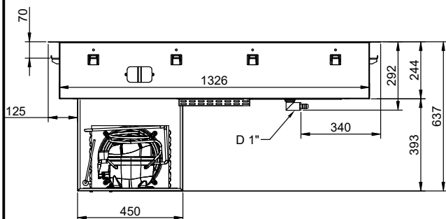
Achterzijde
